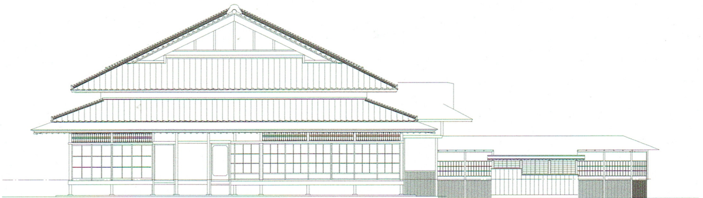
西立面图
