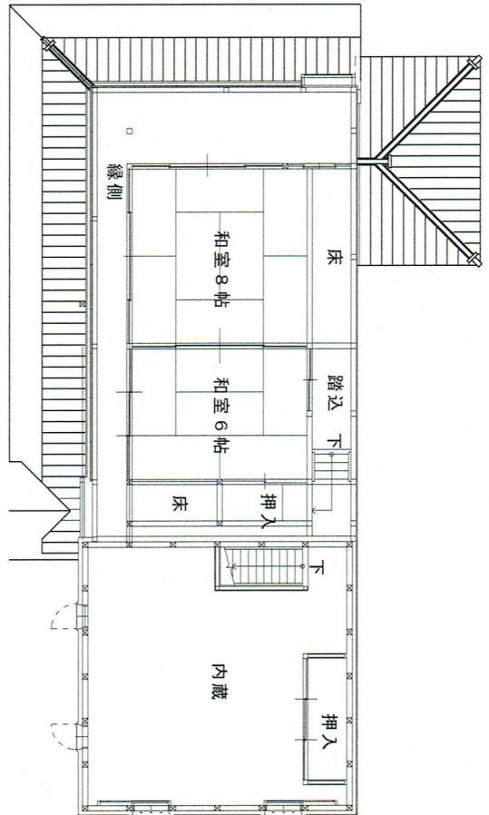
2階平面図
