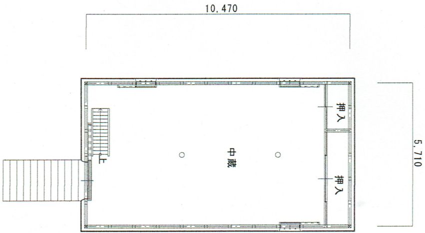
1階平面図
