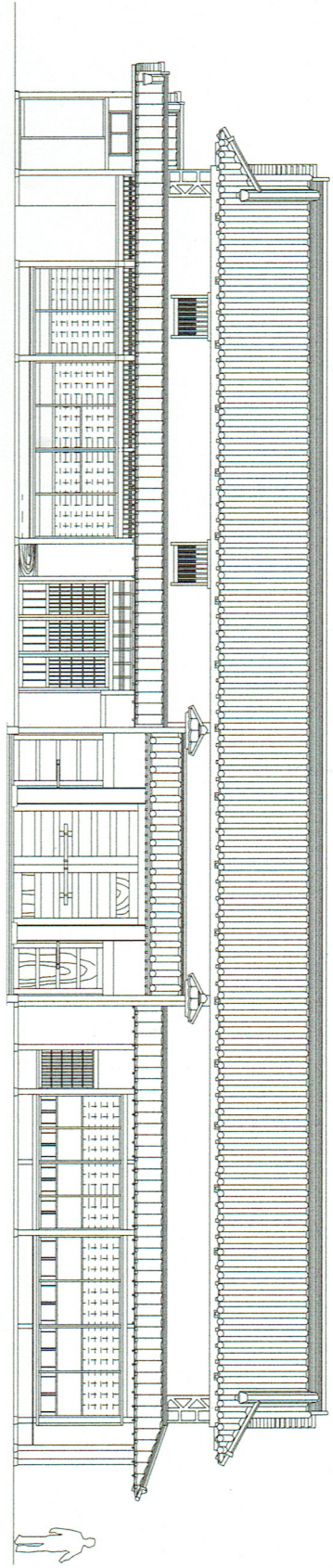
西立面图
